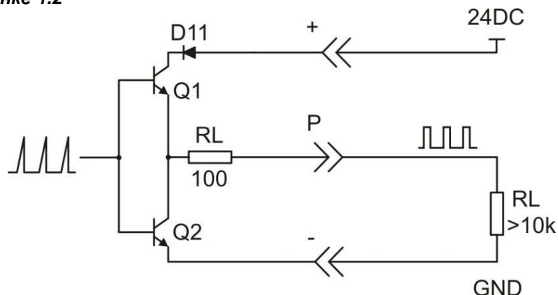
Рисунок 1.2- Схема выходного импульсного каскада
