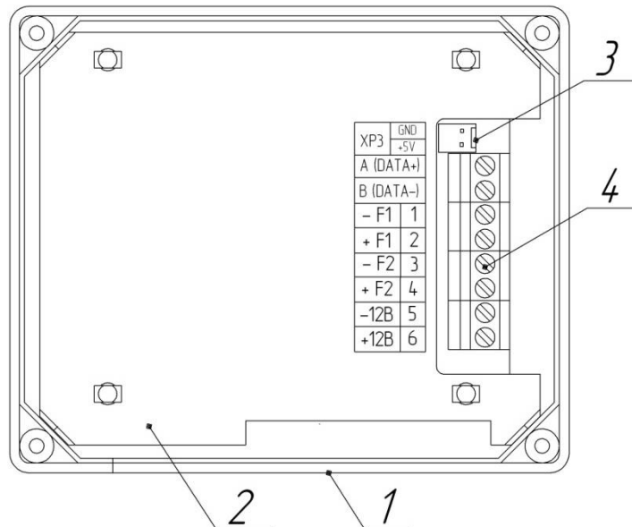
1 - основание корпуса; 2 – фальшпанель; 3 – разъём для подключения к поверочной установке; 4 – колодка клеммная ЭП
