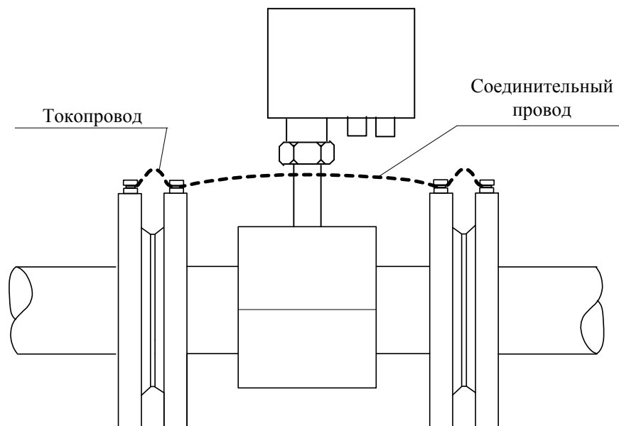
Рисунок 1 – Электрическое соединение фланцев преобразователя
