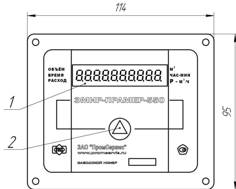
1 - ЖКИ индикатор, 2 – кнопочный переключатель
